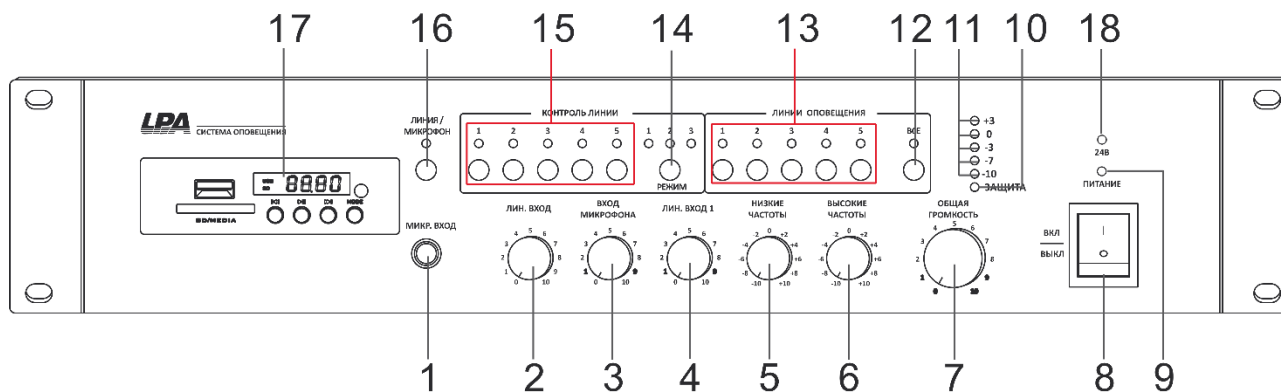
Рис. 1.2. Передняя панель
