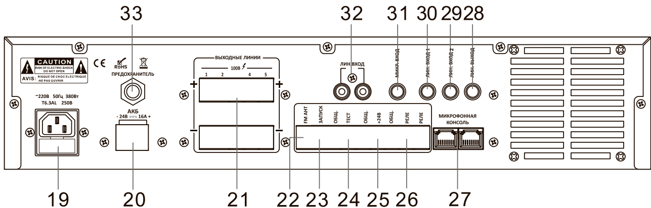
Рис. 1.3. Задняя панель
