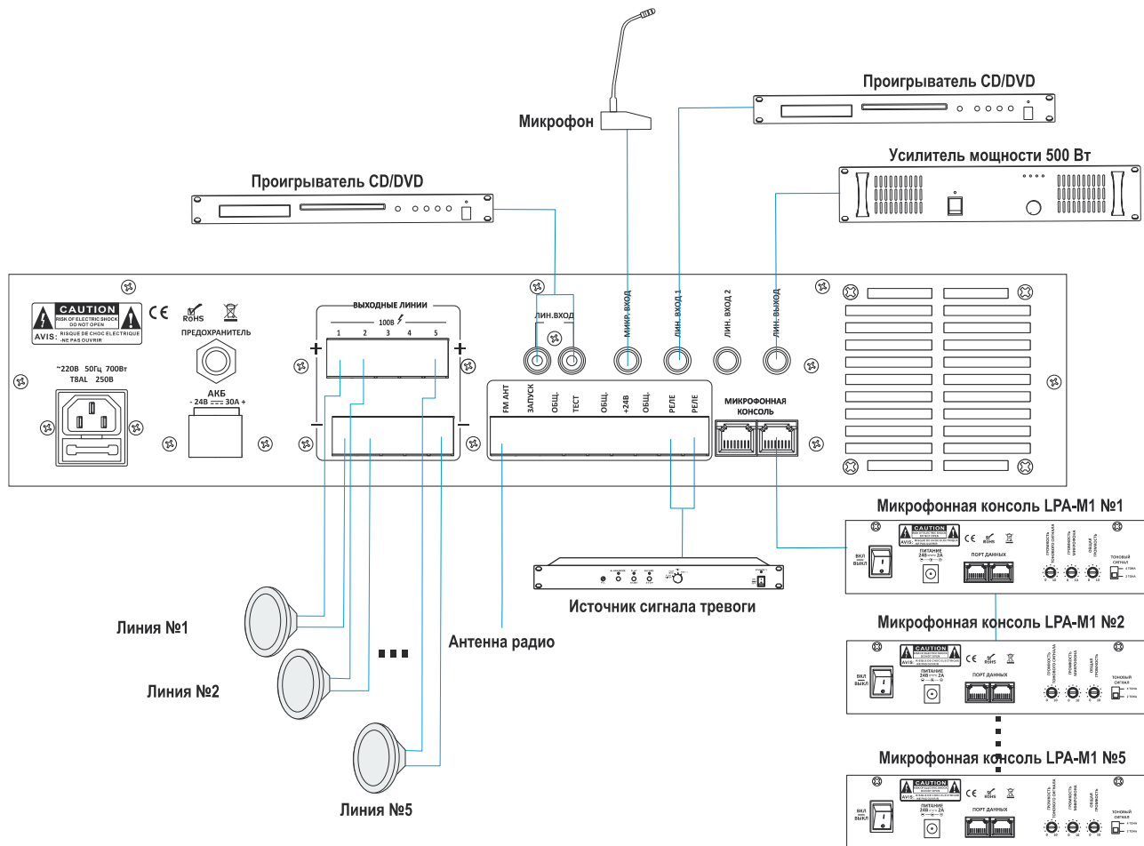
Рис. 2.1. Схема подключения
